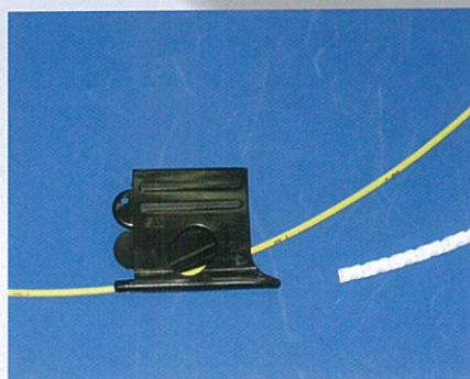
挿入治具に光ケーブルを挟んだ状態
