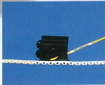
光ケーブルを挿入した状態
